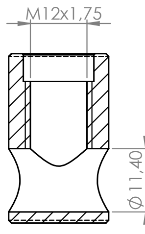
SEÇÃO E-E
