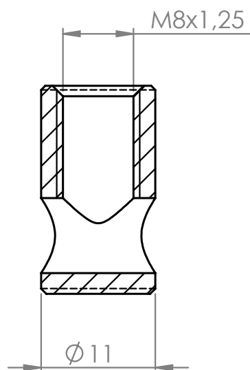
SEÇÃO A-A
