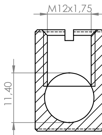
SEÇÃO B-B
