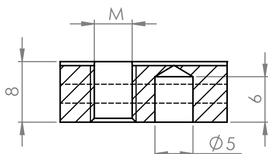
SEÇÃO A-A
