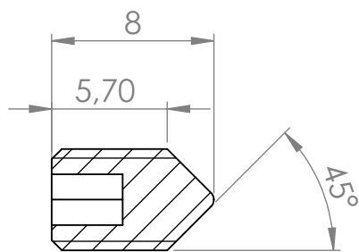
SEÇÃO A-A
