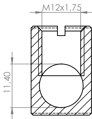
SEÇÃO B-B
