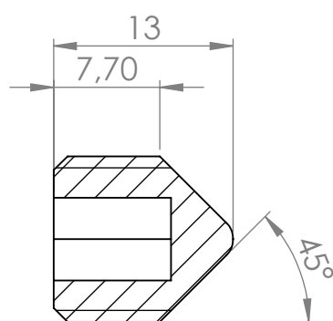
SEÇÃO B-B
