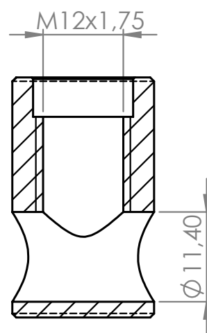
SEÇÃO E-E
