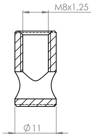
SEÇÃO A-A
