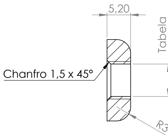
SEÇÃO B-B
