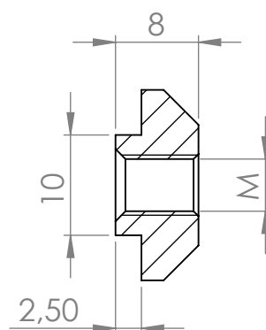
SEÇÃO A-A
