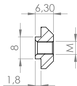
SEÇÃO C-C ESCALA 1 : 1
